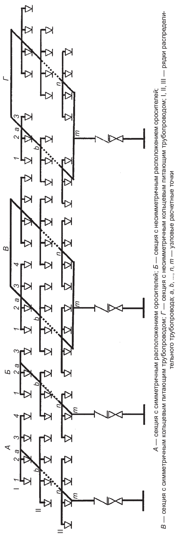
Рисунок В.1 — Схемы распределительной сети спринклерной или дренчерной АУП
