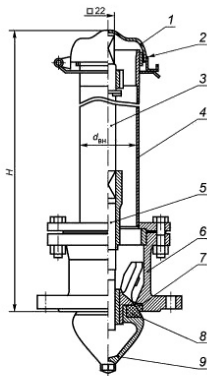
Рисунок А.1 — Гидрант пожарный подземный
