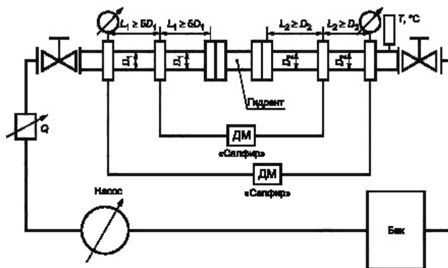
Рисунок В.1 — Схема станда для определения гидравлического сопротивления гидранта
