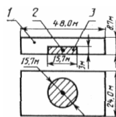
1 - помещение; 2 - аппарат; 3 - взрывоопасная зона Черт. 9
